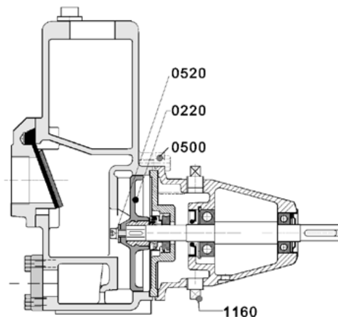
Abb. 11 - Demontage des Laufrades bei Lagerbockgruppe 0, 0+ und 00 (Konstruktion ① und ②)
