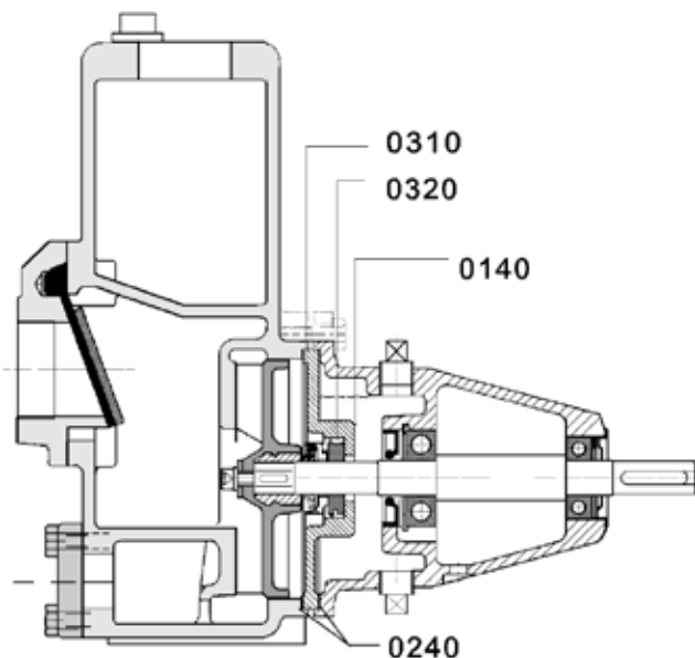
Abb. 12 - Demontage der Gleitringdichtung bei Lagerstuhlgruppe 0 und 00.
